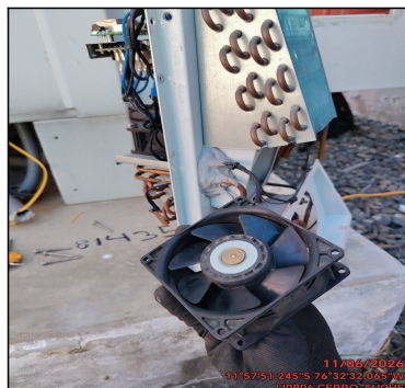
FOTO CORRIENTE REAL EN MOTOR VENTILADOR
