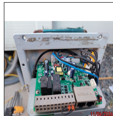
FOTO DE COMPONENTES DE UE (PARTE ELECTRICA)
