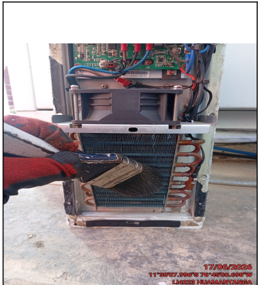
FOTO DE LIMPIEZA Y ESTADO DE SERPENTIN DE UE
