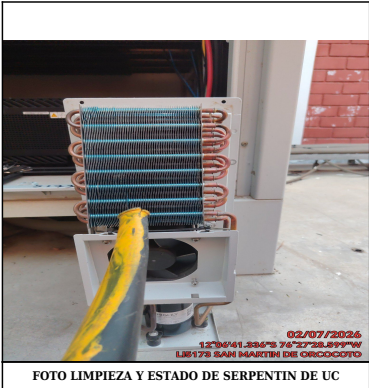
FOTO LIMPIEZA Y ESTADO DE SERPENTIN DE UC
